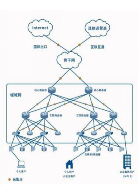
图2：宽带骨干网
