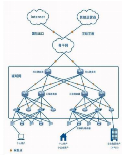
图2：宽带骨干网
